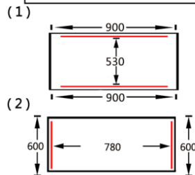
封口架位置標示圖
