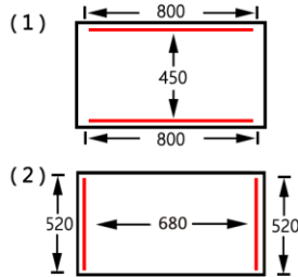
封口架位置標示圖
