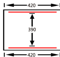
封口架位置標示圖
