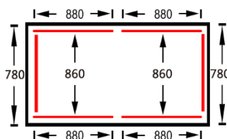
封口架位置標示圖
