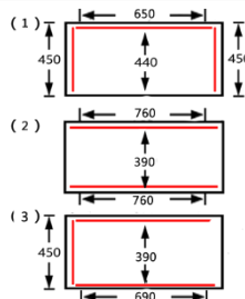
封口架位置標示圖
