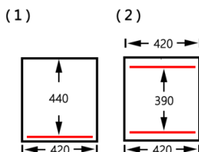
封口架位置標示圖
